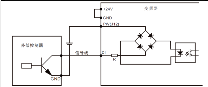
使用外部电源的 NPN 源型连接方式 (注意 J12 去除 PW 与 +24V 之间的跳线)
