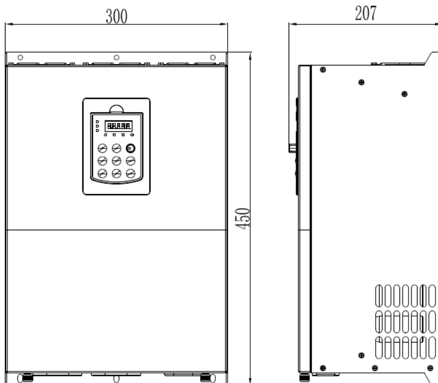
H 系列 T4 版本 30kW—37kW 结构示意图及尺寸
