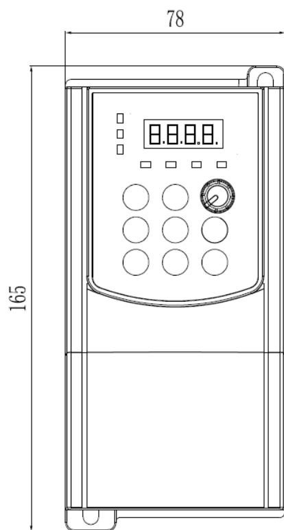
Mini 系列 S2&T4 版本 0.75kW—2.2kW 结构示意图及尺寸
