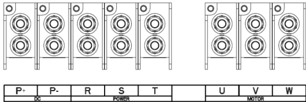
45kW-55kW 主回路端子示意图
