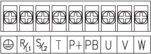
0.75kW-5.5kW 主回路端子示意图
