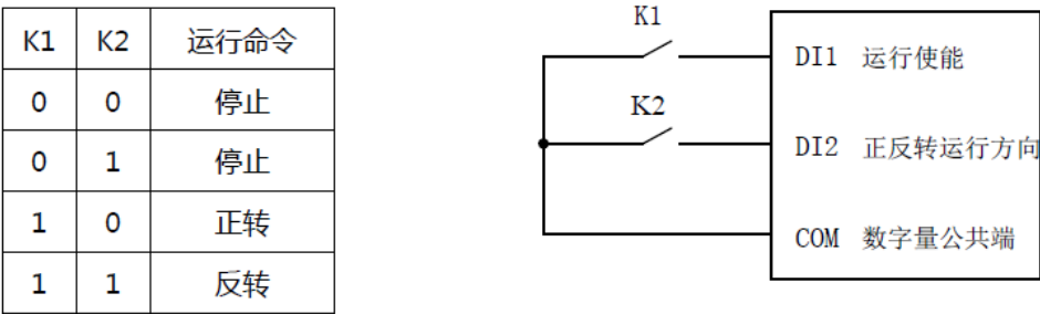
两线式模式 2
