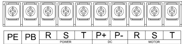
30kW-37kW 主回路端子示意图
