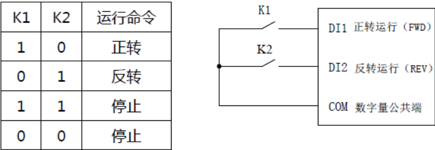
两线式模式 1
