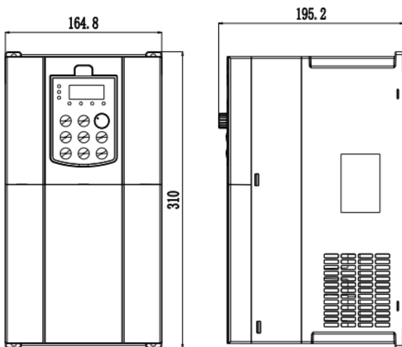
H 系列 T4 版本 15kW—22kW 结构示意图及尺寸
