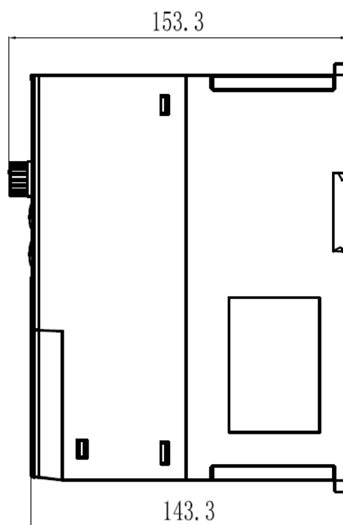
H 系列 T2 版本 2.2kW &H 系列 T4 版本 3.7kW—5.5kW 结构示意图及尺寸
