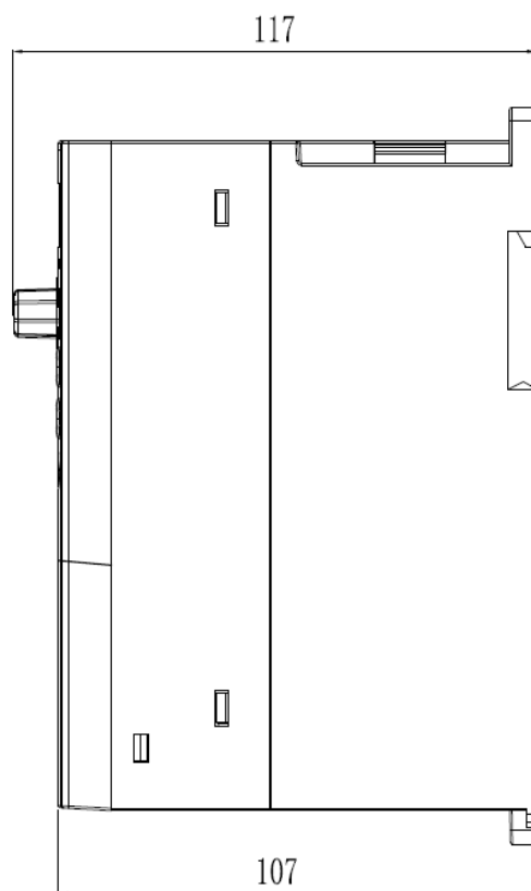
Mini 系列 S2&T4 版本 0.75kW—2.2kW 结构示意图及尺寸
