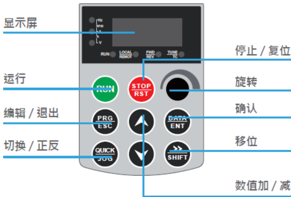
Mini 系列版本键盘示意图
