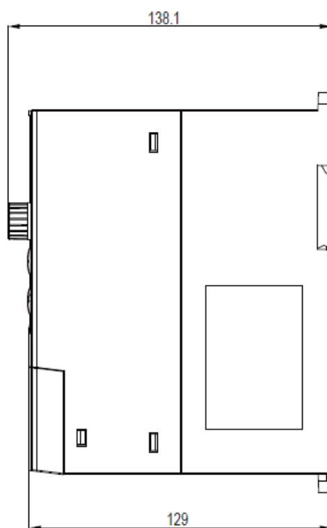
H 系列 T2 版本 0.75kW—1.5kW & H 系列 S2&T4 版本 0.75kW—2.2kW 结构示意图及尺寸
