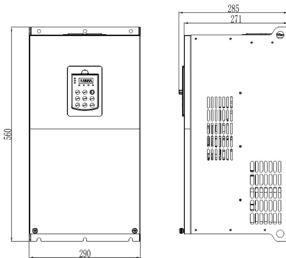
H 系列 T4 版本 45kW—55kW 结构示意图及尺寸
