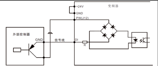
使用外部电源的 PNP 漏型连接方式 (注意 J12 去除 PW 与 +24V 之间的跳线)
