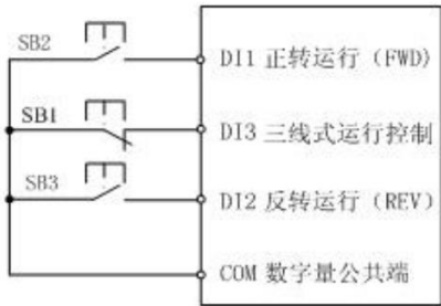
三线式模式 1
