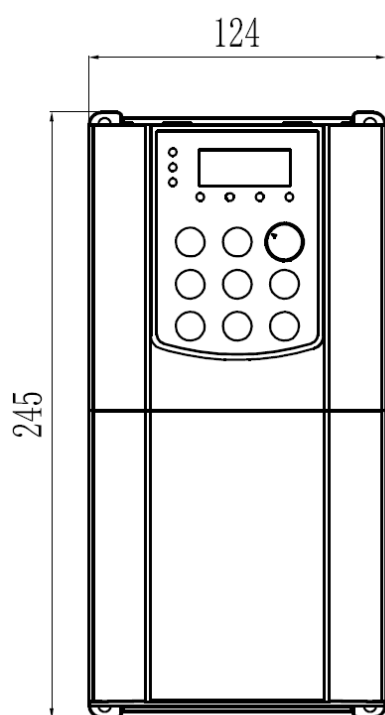
H 系列 S2/T2 版本 3.7kW—5.5kW & H 系列 T4 版本 7.5kW—11kW 结构示意图及尺寸
