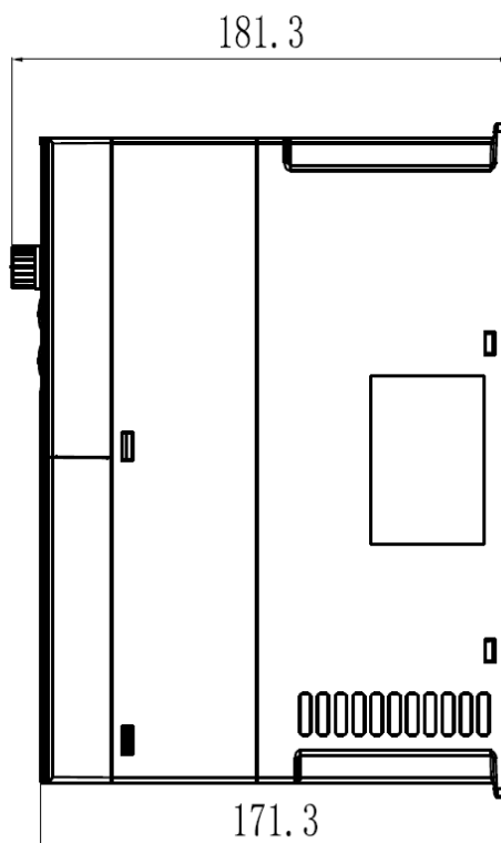
H 系列 S2/T2 版本 3.7kW—5.5kW & H 系列 T4 版本 7.5kW—11kW 结构示意图及尺寸
