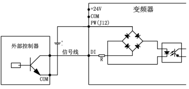
使用外部电源的 NPN 源型连接方式 (注意 J12 去除 PW 与+24V 之间的跳线)
