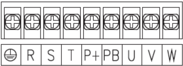
7.5kW-22kW 主回路端子示意图
