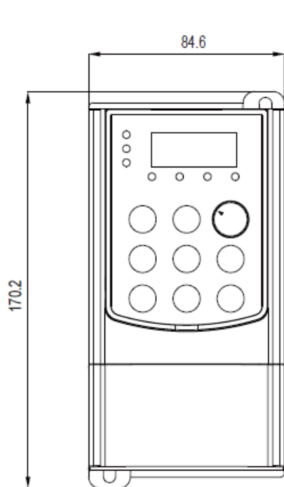
H 系列 T2 版本 0.75kW—1.5kW & H 系列 S2&T4 版本 0.75kW—2.2kW 结构示意图及尺寸
