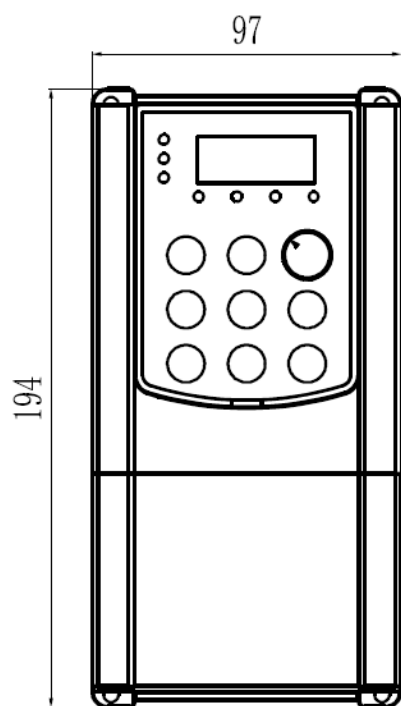
H 系列 T2 版本 2.2kW &H 系列 T4 版本 3.7kW—5.5kW 结构示意图及尺寸
