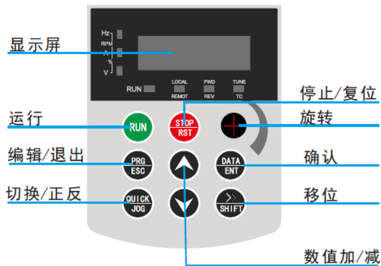
Mini 系列版本键盘示意图
